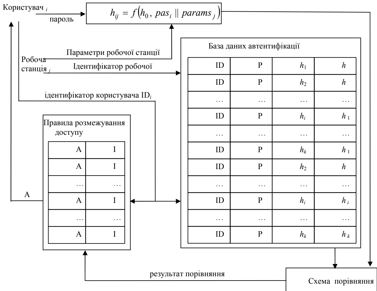
Рисунок 2 – Модифікована схема авторизації користувача з використанням паролів
